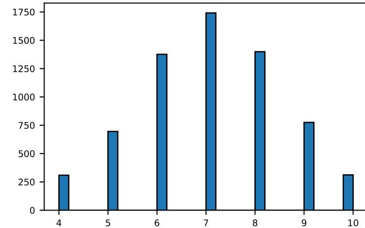
sleep_hours
